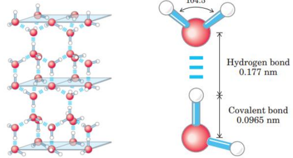
Şekil 6. Buzdaki hidrojen bağları (Nelson, Cox)
